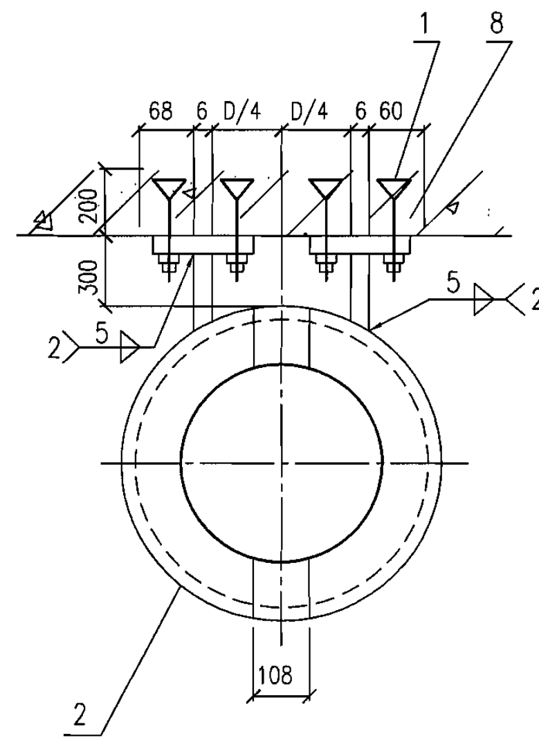
B-B
