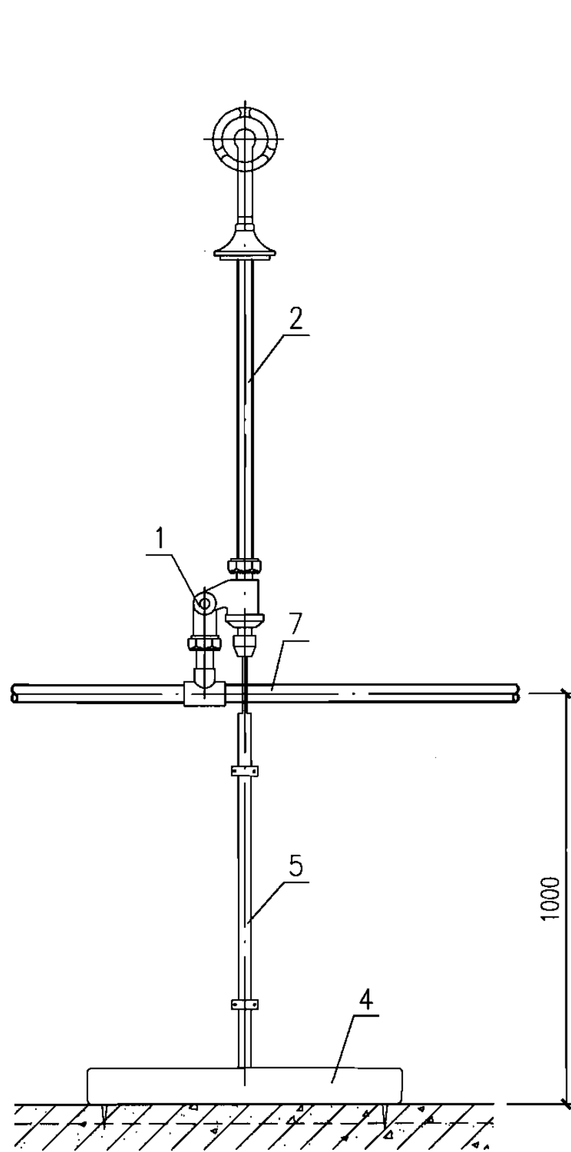
立面图
