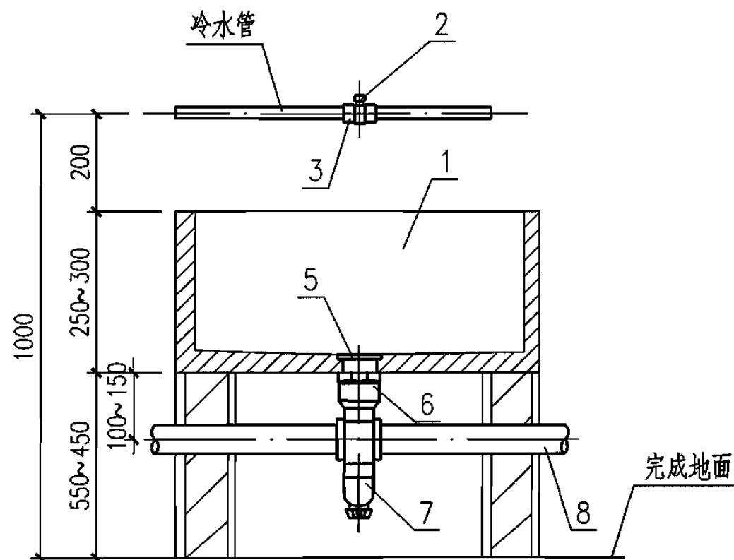
I—I 剖面
