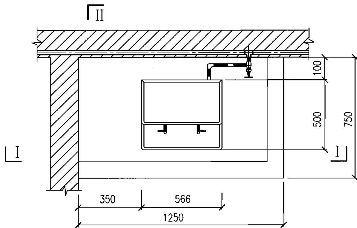
平面图
