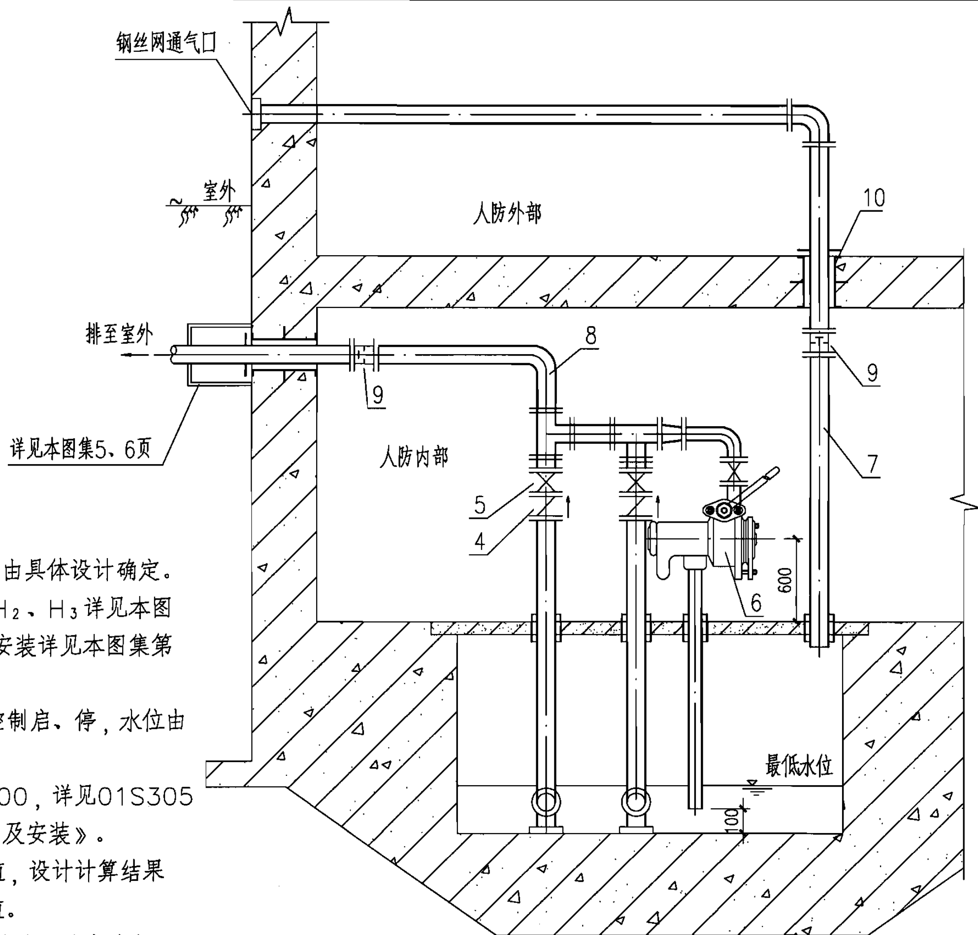
污水提升排水出口图
