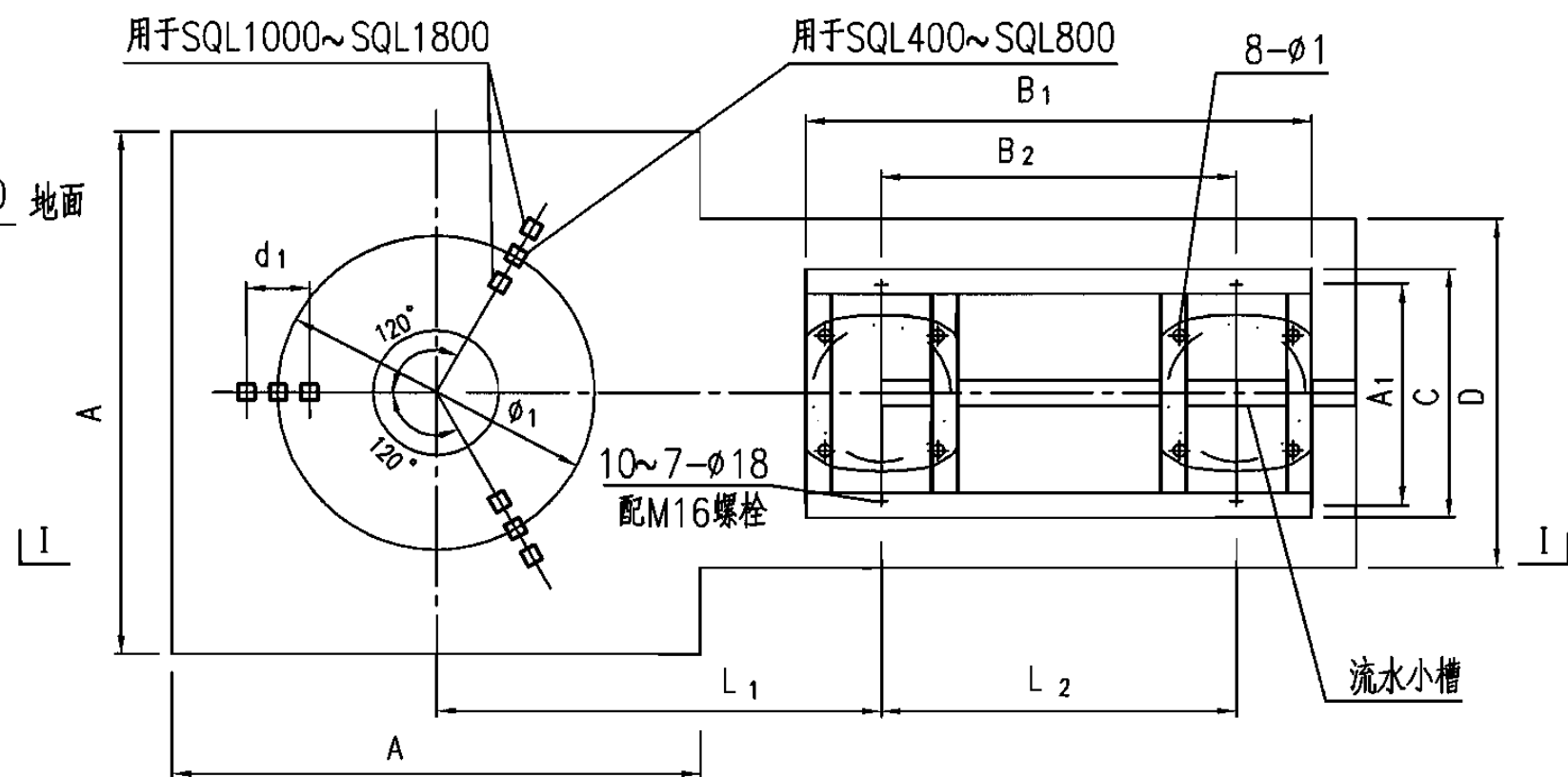
基础平面图
