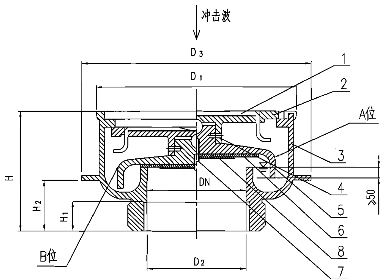
构造图
