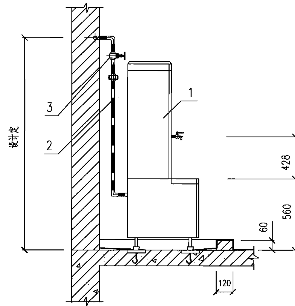
II—II 剖面图
