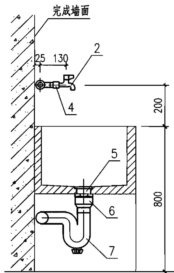
II—II 剖面
