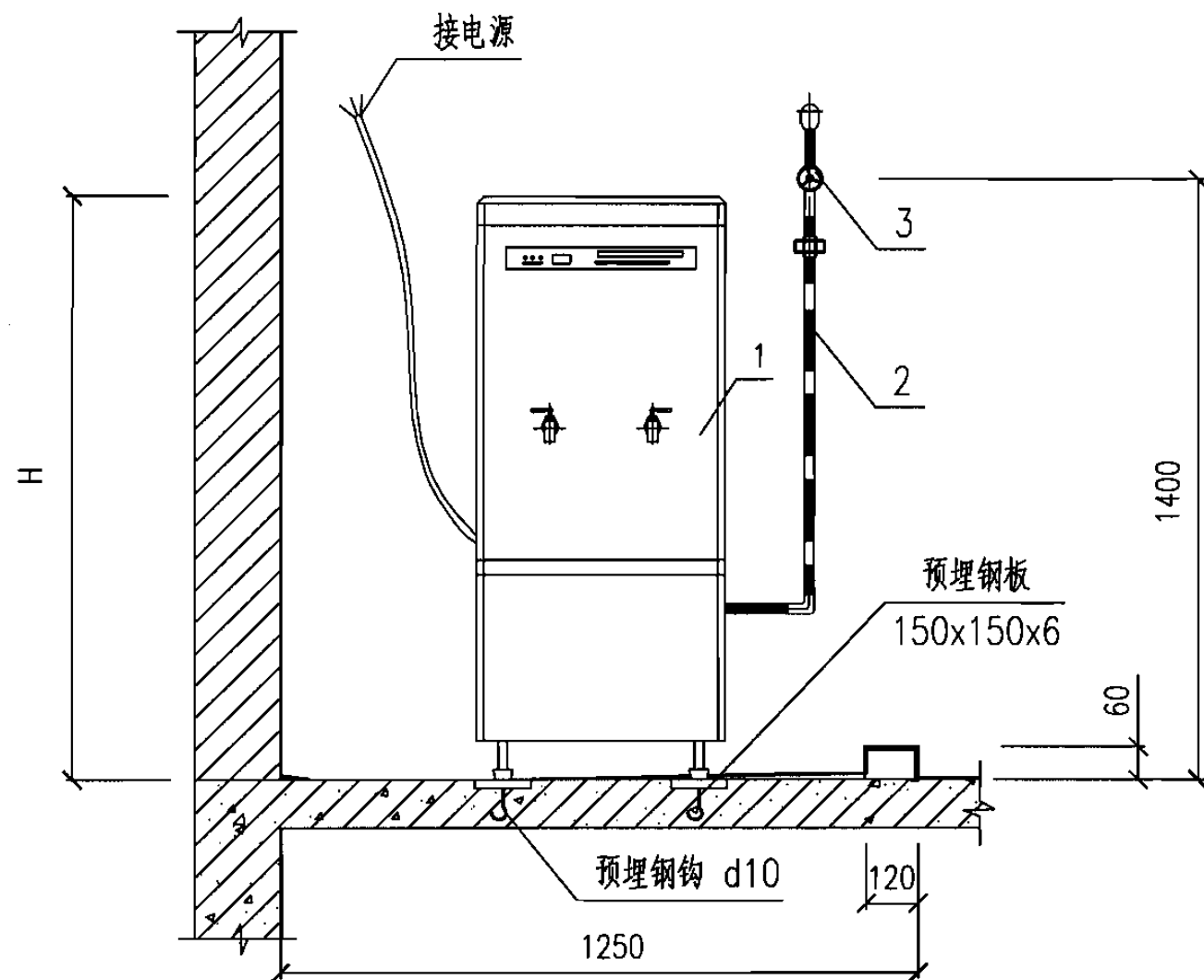
I—I 剖面图
