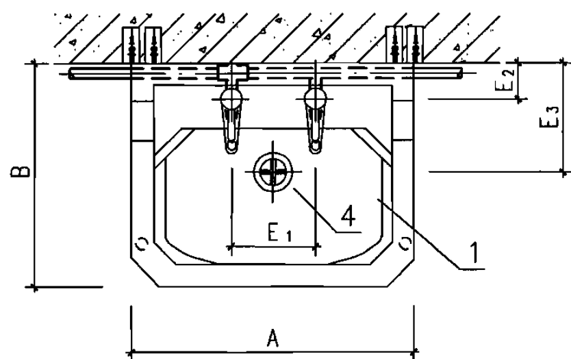
平面图
