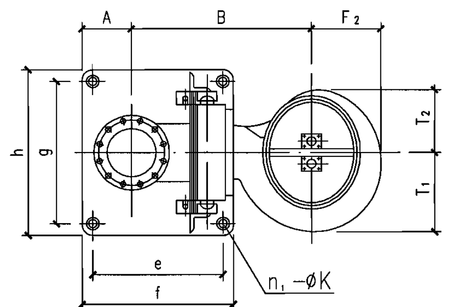
A 向
