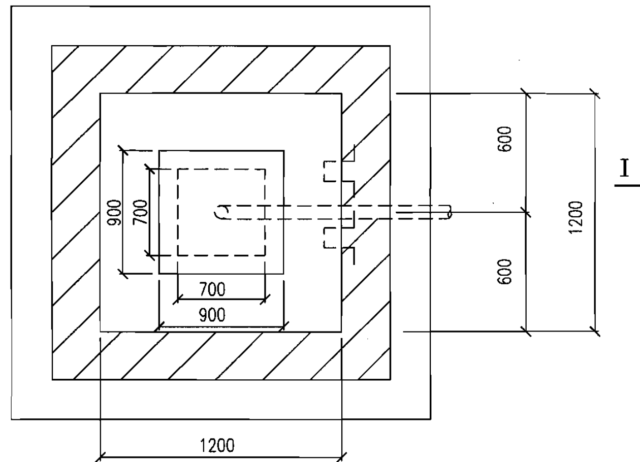
平面图
