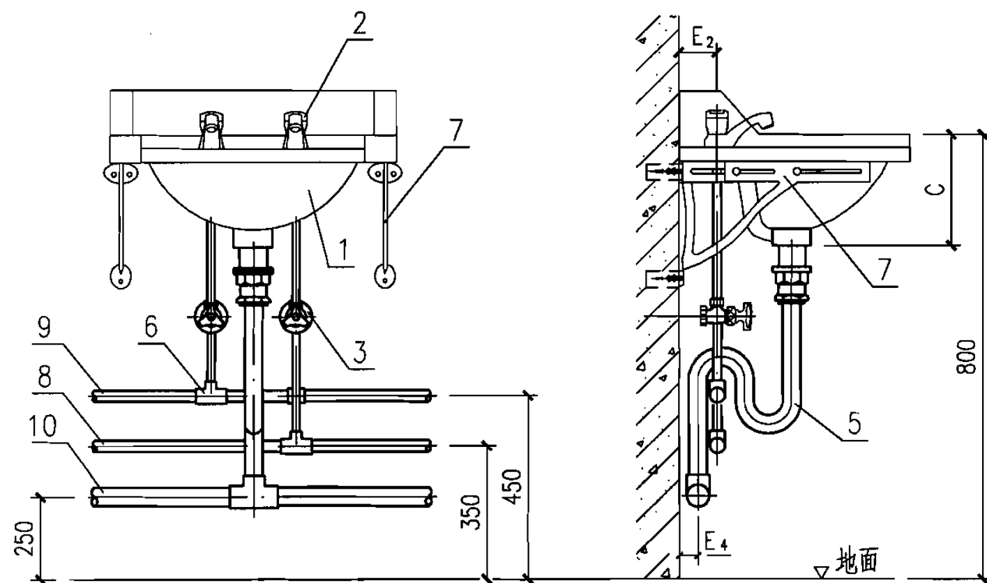
立面图
