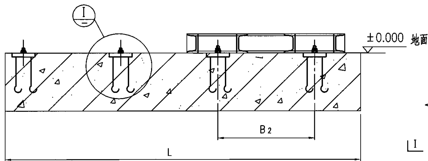
I—I 剖面
