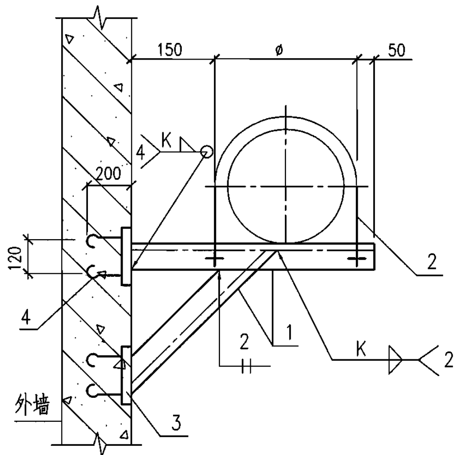
侧面图
