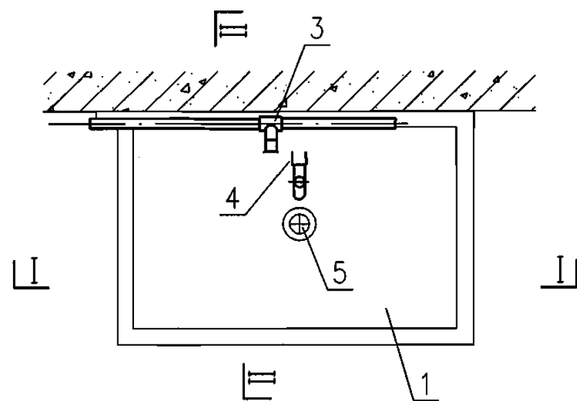
平面图
